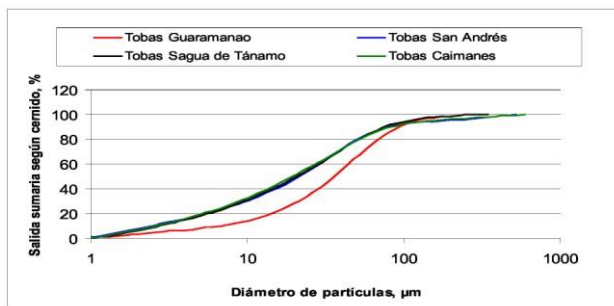
Figura 1. Características de tamaño de las tobas vítreas y zeolitizadas.
