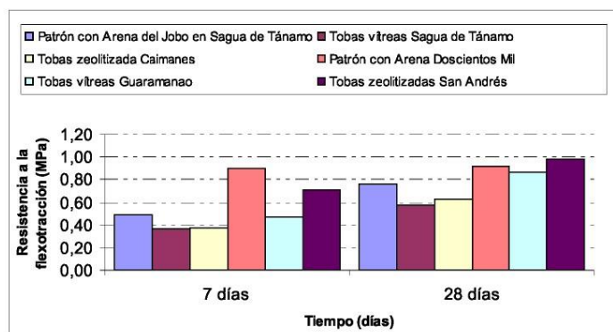
Figura 2. Resistencia a la flexotracción de los morteros patrones y con 15 % de tobas.
