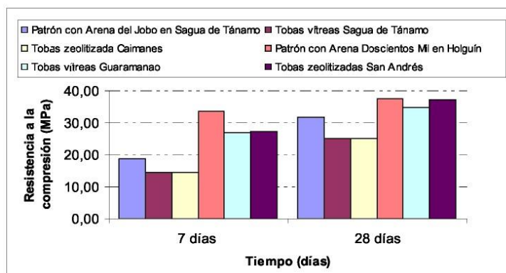
Figura 3. Resistencia a la compresión de los morteros patrones y con 15 % de tobas.
