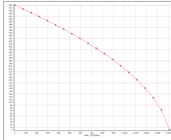
Figura 7. Curva IPR.
