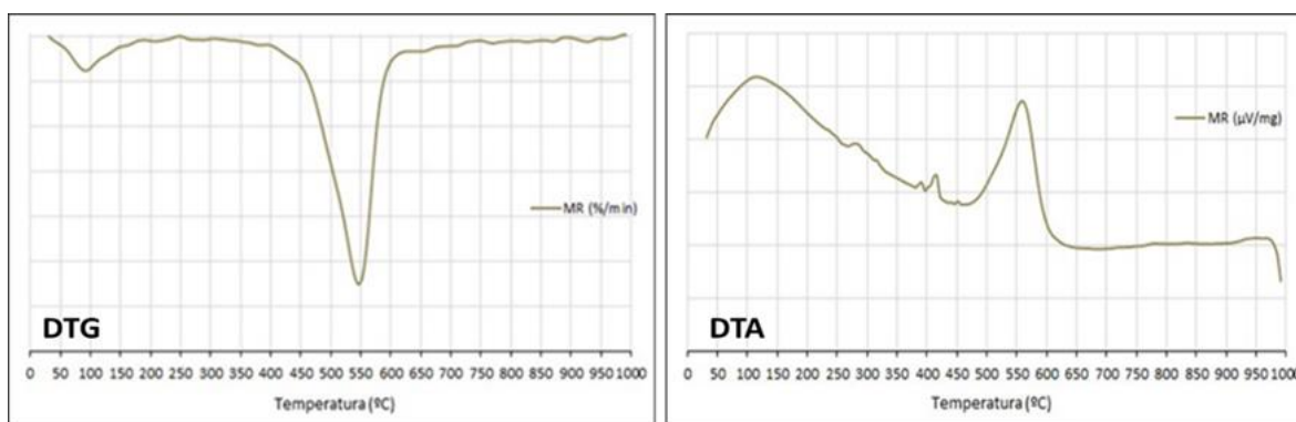
Figura 8. Curvas DTG y DTA mostrando las principales reacciones.
