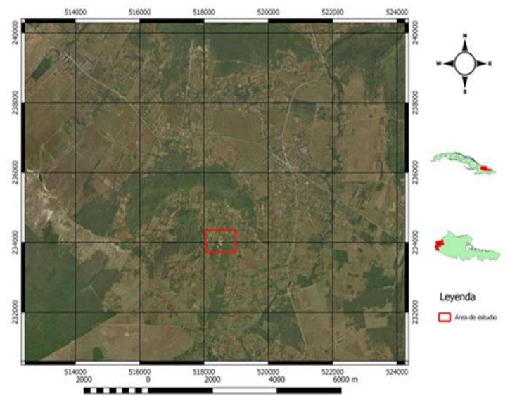
Figura 1. Ubicación geográfica del área de estudio.
