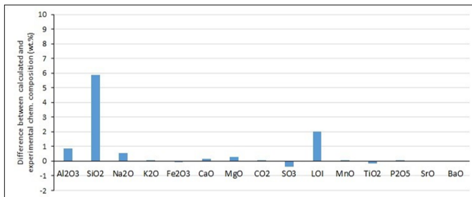
Figura 7. Diferencias entre la composición química estimada con base al Rietveld y la determinada experimentalmente.
