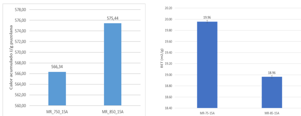
Figura 9. Representación gráfica del calor acumulado (izquierda) y superficie específica (derecha).
