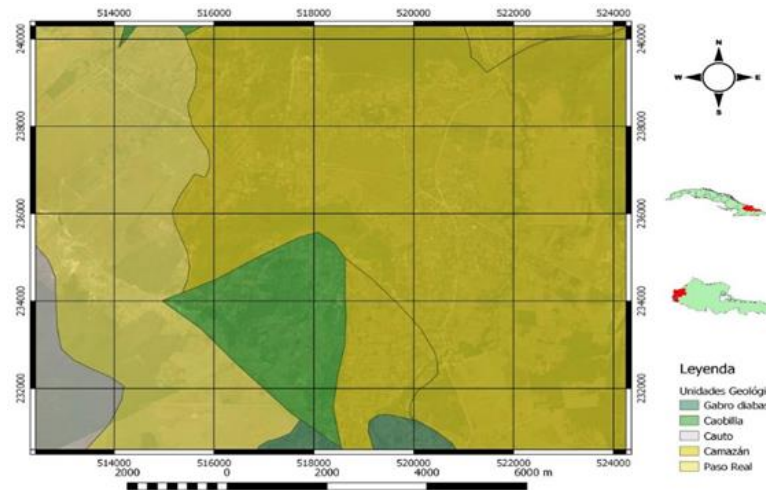
Figura 2. Esquema geológico del área de estudio.
