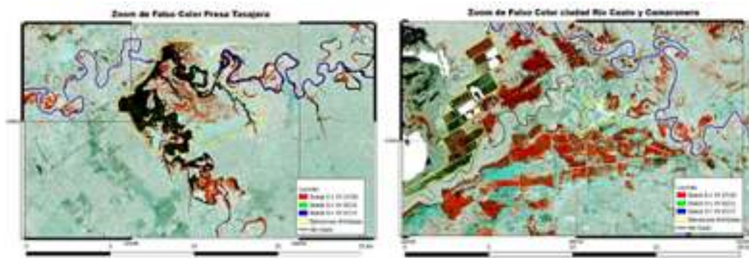
Figura 3. Zoom del Falso Color para zonas de la presa Tasajeras y la ciudad de Río Cauto.
