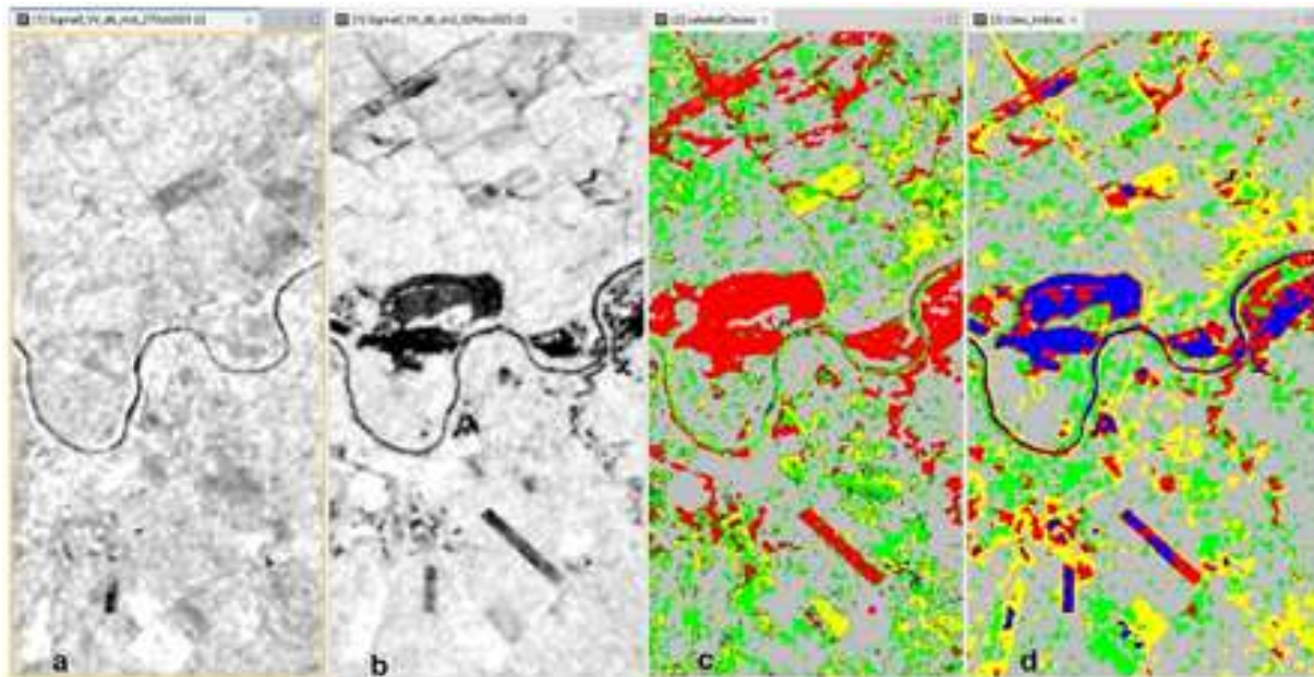
Figura 4. Comparación de imágenes en SNAP con las clasificaciones para un meandro abandonado. a) Antes del paso del huracán (VV 27 de octubre). b) Después del paso del huracán (VV 2 de noviembre). c) Clasificación No Supervisada. d) Clasificación Supervisada.
