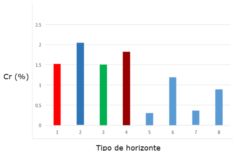
Figura 4. Distribución de los contenidos de cromo, del presente estudio, por tipo de horizonte del perfil laterítico del yacimiento Camarioca Norte.
