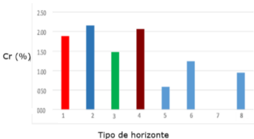
Figura 5. Distribución de los contenidos de cromo en la corteza laterítica por horizonte, según el presente estudio, en el área A-14 del yacimiento Camarioca Norte.
