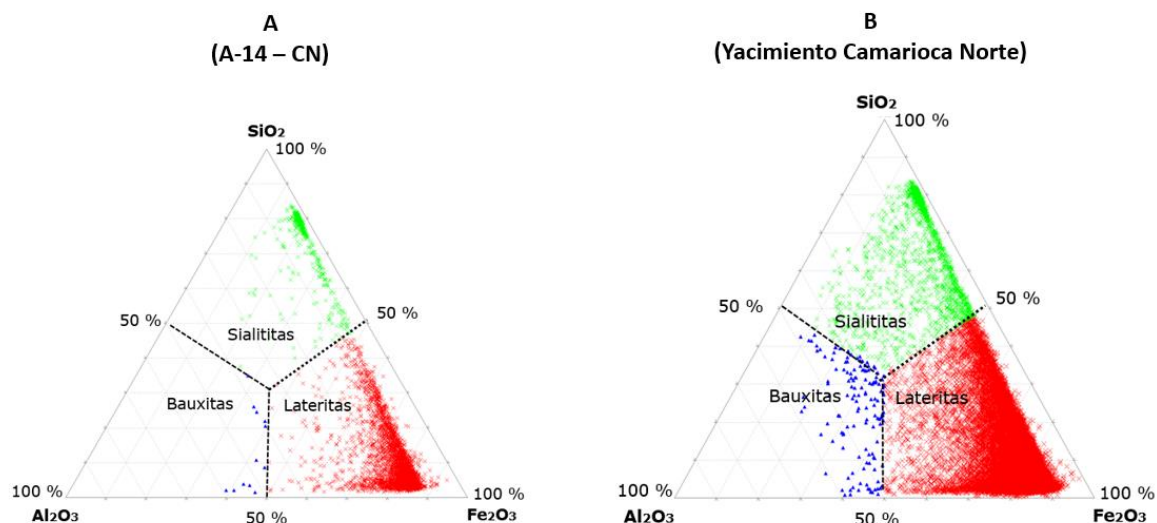
Figura 6. Tipos de cortezas de meteorización del yacimiento Camarioca Norte, según la clasificación propuesta por Lavaut (2023).
