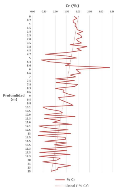
Figura 7. Distribución del contenido de cromo en la corteza laterítica, del presente estudio, en A-14 del yacimiento Camarioca Norte.
