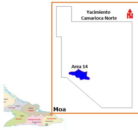
Figura 2. Mapa de ubicación del yacimiento Camarioca Norte.
