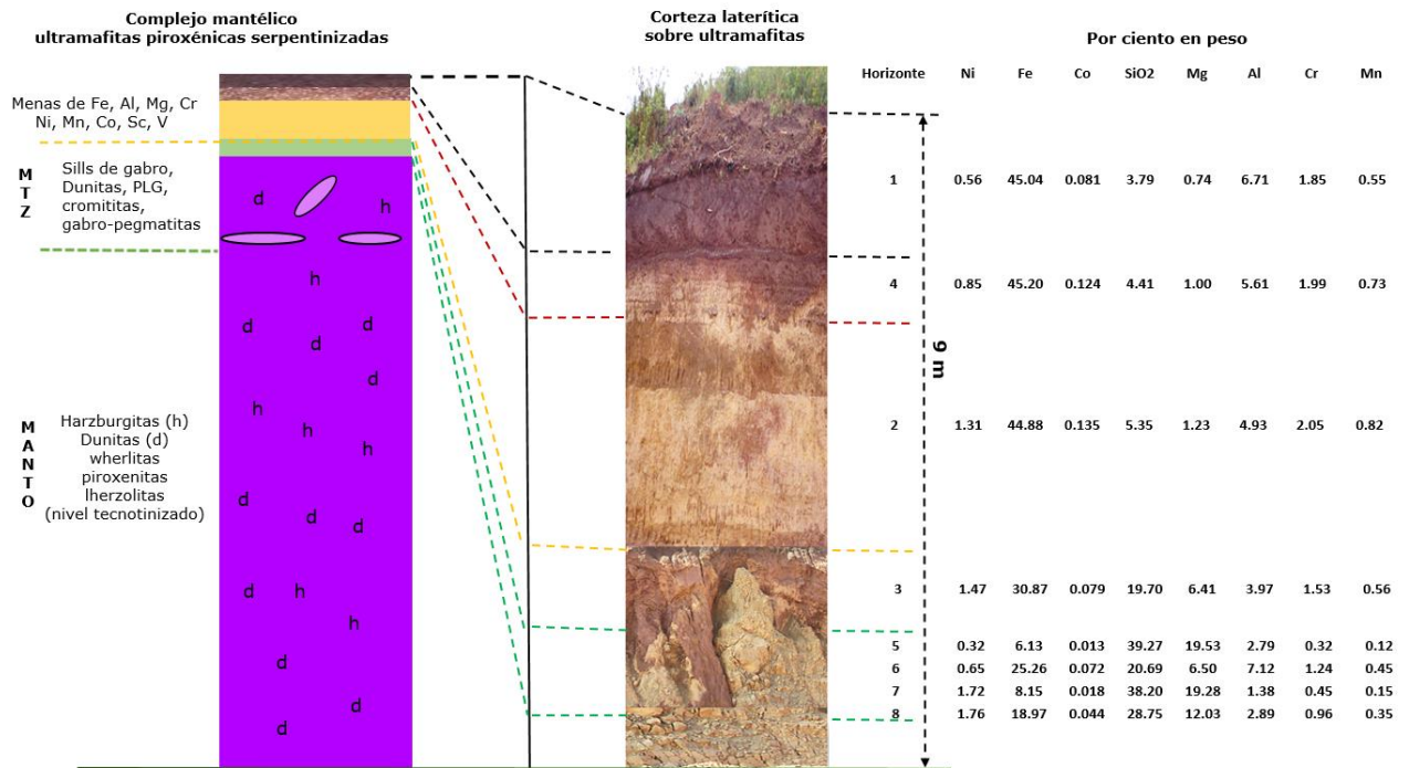
Figura 3. Perfil de la corteza laterítica, tipo óxido, del yacimiento Camarioca Norte, desarrollada sobre el complejo mantélico: ultramafitas piroxénicas serpentinizadas.
