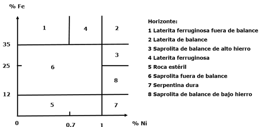
Figura 2. Clasificación de los horizontes del perfil laterítico, tipo óxido, aplicados en la compañía Moa Nickel S.A.
