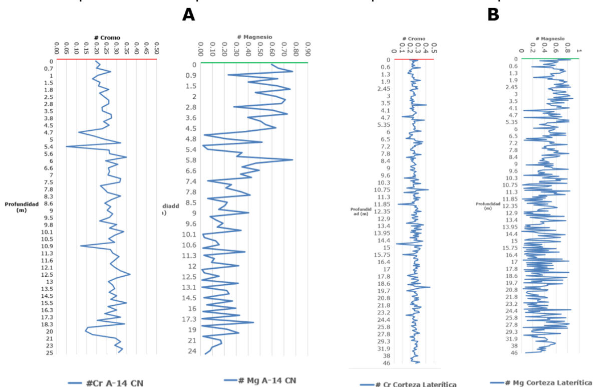
Figura 8. Distribución del número de cromo (# Cr) y número de magnesio (#Mg) (A) área-14 del yacimiento Camarioca Norte y (B) corteza laterítica de níquel y cobalto de Moa.
