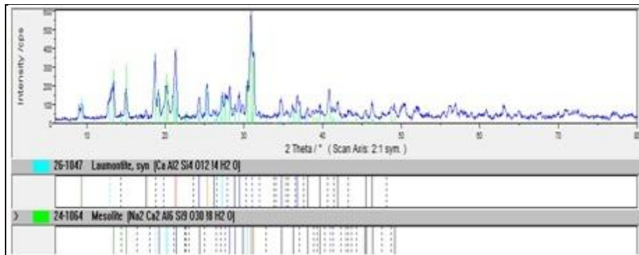
Figura 7. Muestra BZG12 de la región de Goba. Fase principal mesolita con valores principales de d (2,89; 2,86; 2,58). Hay también laumontita, según los picos con valores de d (4,17; 3,51; 3,40).
