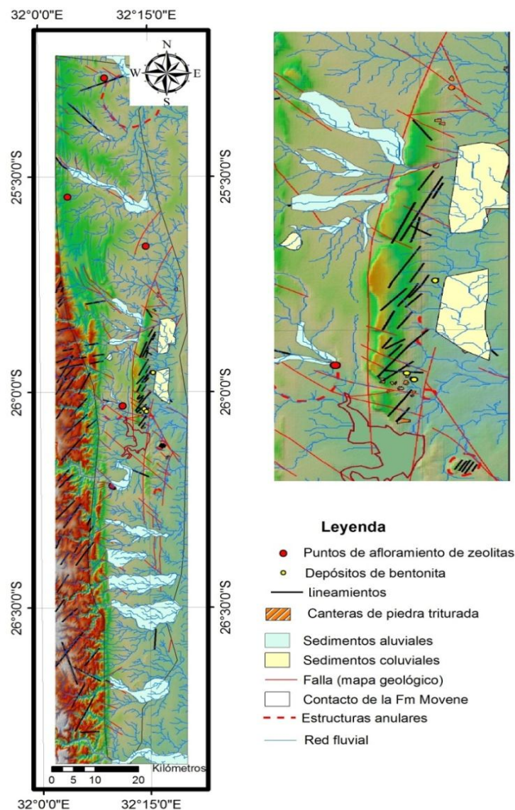
Figura 4. Esquema geológico sobre el modelo de relieve sombreado, que indica los elementos interpretados en las composiciones de falso color y el MDE (sector ampliado a la derecha).
