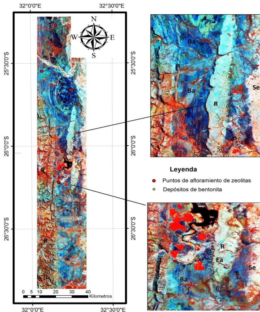
Figura 2. Composición de colores CC5_6_7 donde se diferencian basaltos (Ba), riolitas (R), rocas sedimentarias (Se) y estructuras anulares (Ea).
