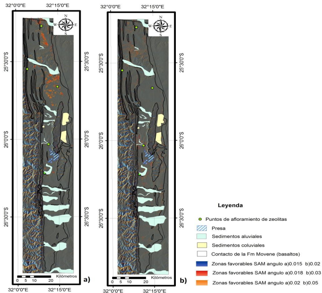
Figura 9. Áreas potenciales para la ocurrencia de zeolitas, a través de la aplicación del SAM, a) usando espectros de referencia (librería espectral) b) usando áreas de entrenamiento (ROI). El mapa base es un modelo de relieve sombreado. Angulo espectral en radianes.
