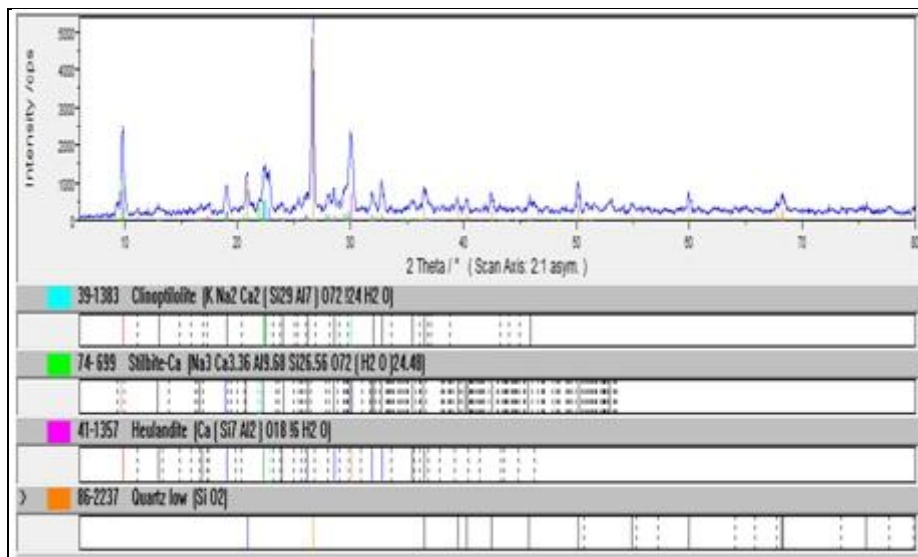
Figura 6. Muestra BMI14 de la región de Goba. Fase principal, cuarzo con valores de d(3,35; 4,25; 1,82) , con clinoptilolita–heulandita, valores de d(8,93; 6,87; 5,12) .
