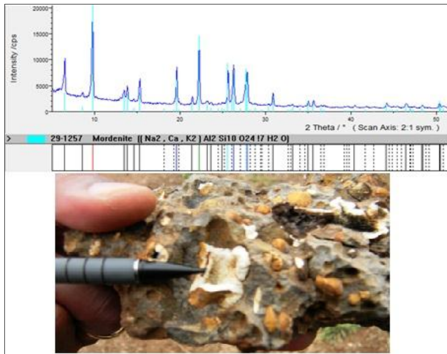
Figura 8. Difractograma de la muestra P-1, cerca de Boane. Las amígdalas del basalto (foto de abajo) están rellenas por mordenita de hábito fibroso y color blanco.
